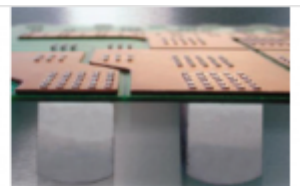
השמה על מעגל עם Busbar
