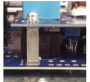
חיבור מעגל למעגל עד 320A
